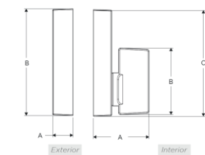
Cilindro Sencillo
